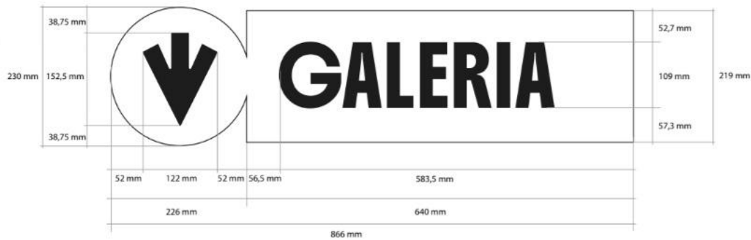
WYMIARY OZNACZEŃ GŁÓWNYCH
